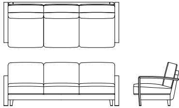
ワイド3Pソファ L08810P WN [W/2200 D/870 H/830 SH/420]
