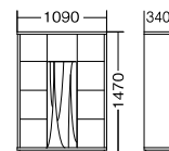
片面木扉(ダンパー付きヒンジ仕様) 開口部サイズ(332×332) ※扉内部3カ所も同じ
