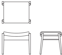
1P スツール X02730Z 【W610 D470 H480 SH450】
