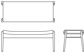
2P ベンチ X02730D 【W1210 D470 H480 SH450】
