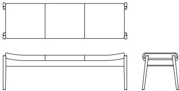
3P ベンチ X02730S 【W1610 D470 H480 SH450】
