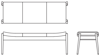
ワイド 2P ベンチ X02730F 【W1410 D470 H480 SH450】
