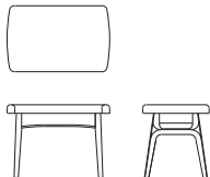
1P スツール X02660Z 【 W620 D400 H440 】
