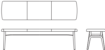
3P ベンチ X02660S 【 W1620 D400 H440 】
