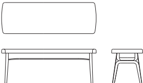
2P ベンチ X02660D 【 W1220 D400 H440 】
