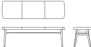
ワイド 2P ベンチ X02660F 【 W1420 D400 H440 】
