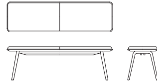
ワイド 2P ベンチ X02611F 【W1400 D400 H445】
