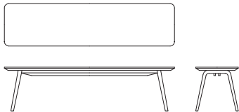
3P ベンチ X02610S 【 W1600 D400 H415 】
