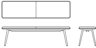
3P ベンチ X02611S 【W1600 D400 H445】
