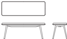
2P ベンチ X02611D 【W1200 D400 H445】
