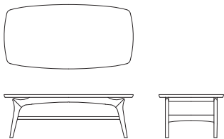
リビングテーブル T04590M 【 W1200 D600 H400(144) 】
