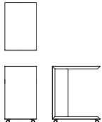
サイドテーブル M04960 Z 【 W295 D450 H537 】
