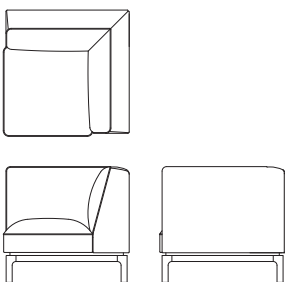
コーナーソファ L09140C 【 W830 D830 H765(140) SH425 】
