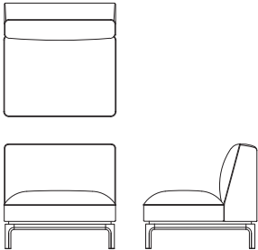
肘無 1P ソファ L09110N 【 W830 D830 H765(140) SH425 】
