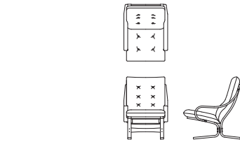
1P ソファ L08670A 【 W660 D860 H940(102) SH450 AH510 】
