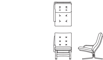
右肘ソファ L08670R 【 W620 D860 H940(102) SH450 AH510 】
