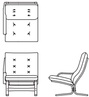
ワイド右肘ソファ L08310M 【 W755 D860 H940(102) SH450 AH510 】
