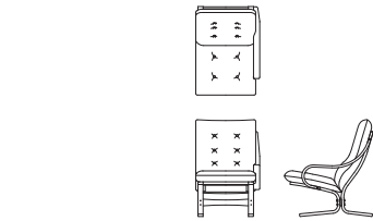
左肘ソファ L08670L 【 W620 D860 H940(102) SH450 AH510 】
