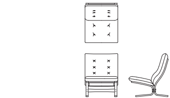
ワイド肘無ソファ L08670U 【 W715 D860 H940(102) SH450 】
