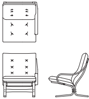
ワイド左肘ソファ L08310H 【 W755 D860 H940(102) SH450 AH510 】
