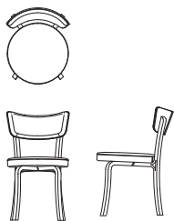
アームレスチェア D03970N 【 W455 D555 H790 SH460 】
