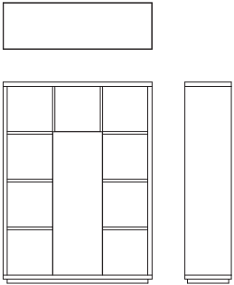
シェルフ B08660Z 【W1090 D340 H1470】 固定棚 (W332:8 枚)
