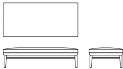
2P ベンチ X02490D 【 W1610 D730 H430(205) 】
