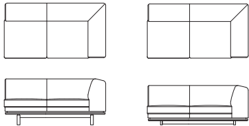
左肘ワイド 2P ソファ L09021L・L09023L【W1560 D850 H710(114) SH420】 L09022L・L09024L【W1560 D850 H610(62) SH320】
