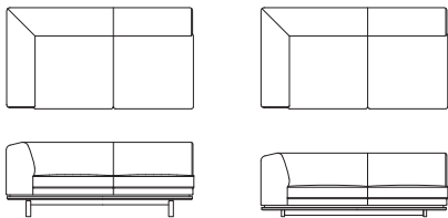
右肘 3P ソファ L09221M・L09223M【W1790 D980 H710(114) SH420】 L09222M・L09224M【W1790 D980 H610(62) SH320】
