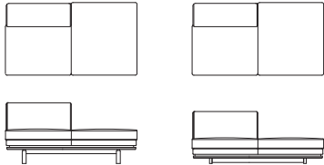
右肘無 3P ソファ (1P 背無) L09011R・L09013R【W1530 D850 H710(114) SH420】 L09012R・L09014R【W1530 D850 H610(62) SH320】
