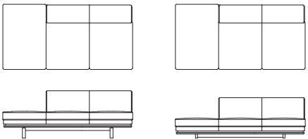
左肘無ワイド 3P ソファ (1P 背無) L09211H・L09213H【W1950 D980 H710(114) SH420】 L09212H・L09214H【W1950 D980 H610(62) SH320】
