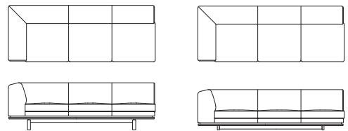
右肘ワイド 3P ソファ L09031R・L09033R 【W2210 D850 H710(114) SH420】 L09032R・L09034R 【W2210 D850 H610(62) SH320】
