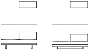
左肘無 3P ソファ (1P 背無) L09211L・L09213L【W1530 D980 H710(114) SH420】 L09212L・L09214L【W1530 D980 H610(62) SH320】
