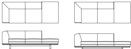
右肘ワイド 3P ソファ (1P 背無) L09031M・L09033M 【W2210 D850 H710(114) SH420】 L09032M・L09034M 【W2210 D850 H610(62) SH320】
