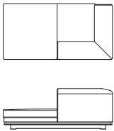
左肘シェーズロング L09001H・L09003H【W850 D1650 H710(114) SH420】 L09002H・L09004H【W850 D1650 H610(62) SH320】
