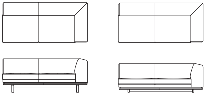
左肘 3P ソファ L09021H・L09023H【W1790 D850 H710(114) SH420】 L09022H・L09024H【W1790 D850 H610(62) SH320】
