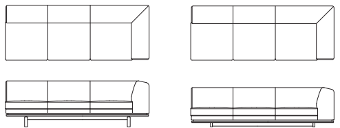
左肘ワイド 3P ソファ L09031L・L09033L 【W2210 D850 H710(114) SH420】 L09032L・L09034L 【W2210 D850 H610(62) SH320】
