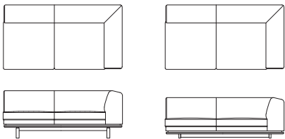
左肘 3P ソファ L09221H・L09223H【W1790 D980 H710(114) SH420】 L09222H・L09224H【W1790 D980 H610(62) SH320】
