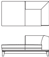
右肘シェーズロング L09001M・L09003M【W850 D1650 H710(114) SH420】 L09002M・L09004M【W850 D1650 H610(62) SH320】
