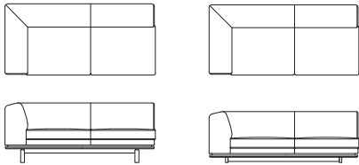
右肘 3P ソファ L09021M・L09023M【W1790 D850 H710(114) SH420】 L09022M・L09024M【W1790 D850 H610(62) SH320】
