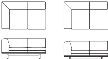
右肘ワイド 2P ソファ L09221R・L09223R【W1560 D980 H710(114) SH420】 L09222R・L09224R【W1560 D980 H610(62) SH320】
