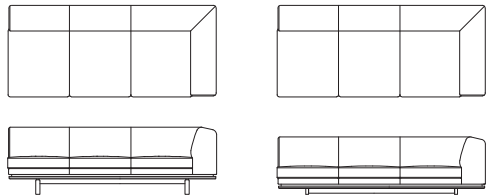
左肘ワイド 3P ソファ L09231L・L09233L【W2210 D980 H710(114) SH420】 L09232L・L09234L【W2210 D980 H610(62) SH320】
