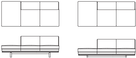
左肘無ワイド 3P ソファ (1P 背無) L09011H・L09013H【W1950 D850 H710(114) SH420】 L09012H・L09014H【W1950 D850 H610(62) SH320】
