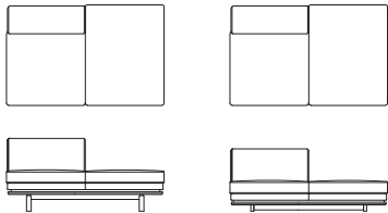
右肘無 3P ソファ (1P 背無) L09211R・L09213R【W1530 D980 H710(114) SH420】 L09212R・L09214R【W1530 D980 H610(62) SH320】
