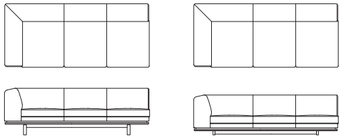
右肘ワイド 3P ソファ L09231R・L09233R【W2210 D980 H710(114) SH420】 L09232R・L09234R【W2210 D980 H610(62) SH320】
