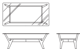
リビングテーブル T04160M 【 W1200 D600 H400(183) 】
