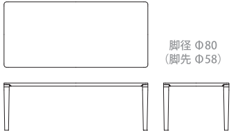
ダイニングテーブル R03970G 【 W2200(2040) D1000(840) H720(675) 】
