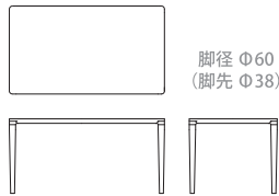
ダイニングテーブル R03970C 【 W1500(1380) D850(730) H720(675) 】
