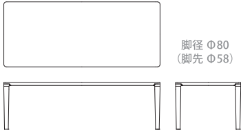
ダイニングテーブル R03970R 【 W2400(2240) D1000(840) H720(675) 】
