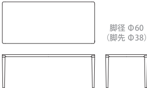
ダイニングテーブル R03970B 【 W2000(1880) D900(780) H720(675) 】
