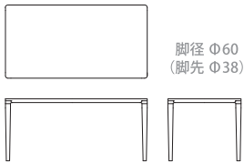
ダイニングテーブル R03970X 【 W1650(1530) D850(730) H720(675) 】
