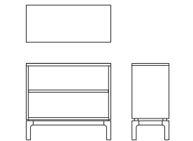
シェルフ B09160Z 【 W800 D350 H720(140) 】
