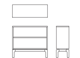
シェルフ B09161Z 【 W800 D290 H720(140) 】
