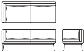
右肘 3P ソファ L08740M 【W1860 D725 H735(205) SH430】
