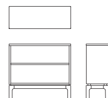
シェルフ B09161Z 【W800 D290 H720(140)】
