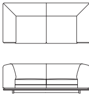
両肘ワイド 2P ソファ L09021F・L09023F【W1810 D850 H710(114) SH420】 L09022F・L09024F【W1810 D850 H610(62) SH320】
