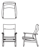
リクライニングチェア P04870A 【W660 D740~945 H970~915(170) SH450 AH610】
