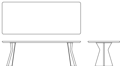
ダイニングテーブル R05640G 【 W2200(1450/1150/850) D900 H710(670) 】
