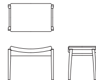
1P スツール X02140Z 【W610 D380 H460 SH430】
