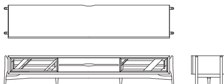
TV ボード B08803Z 【W2310(2200) D450 H400(73)】 □可動棚 (W616: 2 枚)
