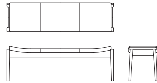
ワイド 2P ベンチ X02140F 【W1410 D380 H460 SH430】
