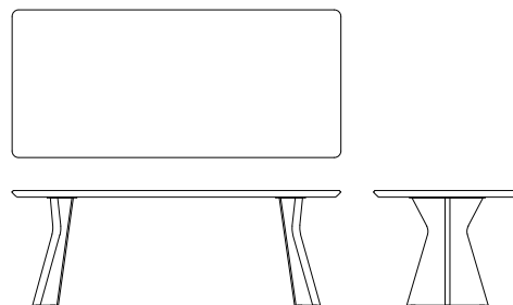
ダイニングテーブル R05640B 【 W2000(1250/950) D900 H710(670) 】
