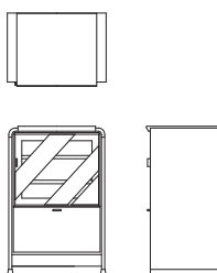
オーディオボード B08455R 【 W593(577) D440 H900(60) 】 □可動棚 (W489: 2 枚)
