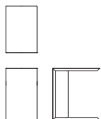
サイドテーブル M04950Z 【 W295 D450 H500 】
