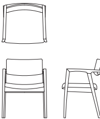
ワイドアームチェア D03780B 【W580 D525 H765 SH435 AH640】
