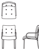
アームチェア D04580A 【W550 D635 H860 SH450 AH585】
