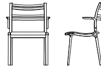
ワイドセミアームチェア D04270E 【W585 D530 H830 SH440 AH640】
