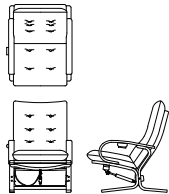
リクライニングチェア P04840A 【 W700 D870~1070 H965~820 SH445 AH550 】
