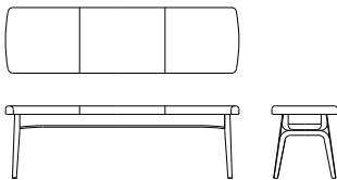
ワイド 2P ベンチ X02660F 【W1420 D400 H440】
