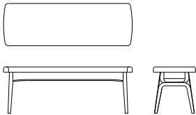
2P ベンチ X02660D 【 W1220 D400 H440 】
