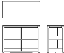
シェルフ S02210M 【 W1000 D450 H720 】
