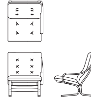
ワイド左肘ソファ L08670H 【W755 D860 H940(102) SH450 AH510】
