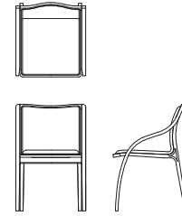
セミアームチェア D04230N 【W510 D545 H780 SH445】
