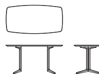
LD テーブル R04121Y 【 W1200(550) D600(575) H600(575) 】
