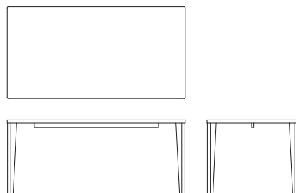
ダイニングテーブル R04460X 【 W1650(1440) D850(640) H700(670) 】
