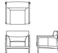
1P ソファ L08550A 【W880 D810 H780(134) SH410】
