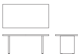
ダイニングテーブル R04091X 【W1650(1300/1150/1000) D850 H700(658)】
