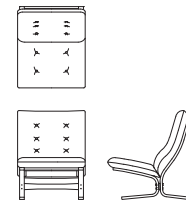
ワイド肘無ソファ L08310U 【W715 D860 H940(102) SH450】
