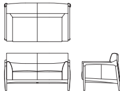
2P ソファ L08550D 【W1380 D810 H780(134) SH410】
