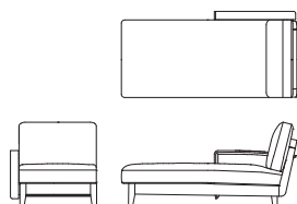
右肘シェーズロング L09040R 【W835 D1700 H830(125) SH420】
