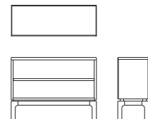
シェルフ B09171Z 【W800 D290 H590(140)】
