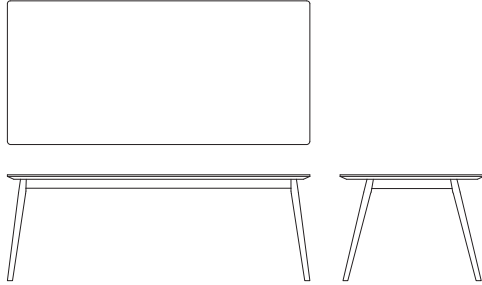
ダイニングテーブル R04450B 【 W2000(1751) D950(532) H700(670) 】
