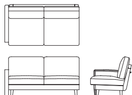
右肘ワイド 2P ソファ L08810R 【W1580 D870 H830(125) SH420】
