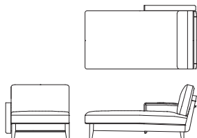
右肘ワイドシェーズロング L09040M 【W970 D1700 H830(125) SH420】
