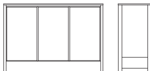
サイドボード B08430Z 【W1320 D445 H900】 □可動棚 (W819:2枚) (W408:2枚)
