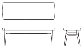
2P ベンチ X02660D 【W1220 D400 H440】
