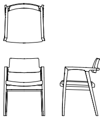
アームチェア D04520A 【W535 D515 H750 SH435 AH640】
