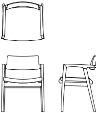
ワイドアームチェア D04520B 【W580 D525 H755 SH435 AH640】
