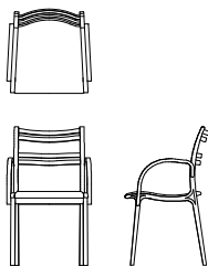
アームチェア D04270A 【W505 D505 H830 SH440 AH640】
