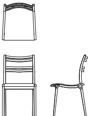
アームレスチェア D04270N 【W465 D505 H830 SH440】
