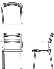
セミアームチェア D04270T 【W510 D505 H830 SH440 AH640】
