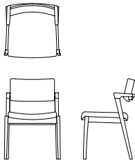
アームレスチェア D03780N 【W535 D515 H765 SH435 AH630】
