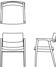
ワイドアームチェア D03780B 【W580 D525 H765 SH435 AH640】
