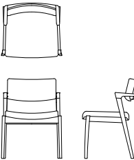
ワイドアームレスチェア D03780U 【W580 D525 H765 SH435 AH630】
