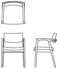
アームチェア D03780A 【W535 D515 H765 SH435 AH640】
