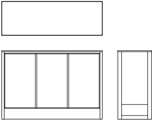
サイドボード B08430Z 【 W1320 D445 H900 】 可動棚 (W819:2 枚) (W408:2 枚)
