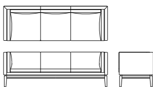
両肘ワイド 3P ソファ L08760P 【W2200 D725 H735(205) SH430】
