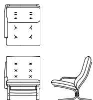
ワイド右肘ソファ L08670M 【W755 D860 H940(102) SH450 AH510】
