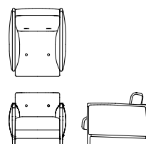
1P ソファ L09180A 【W840 D1015 H805(125) SH440】
