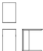
サイドテーブル M04950 Z 【 W295 D450 H500 】
