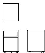
ワゴン (抽斗2段) S02190Z 【W360 D400 H550】
