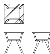
サイドテーブル T04160S 【W450 D450 H500(257)】
