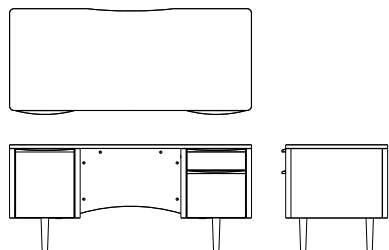
デスク S02161Z 【W1600(760) D700 H720(695)】
