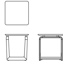
サイドテーブル T04720S 【W500 D500 H552】
