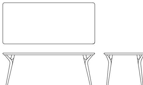
ダイニングテーブル R04540B 【W2000(1485) D900(530) H710(670)】
