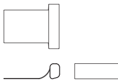
ヘッドレスト 001500Z 【W600 D740 H140】
