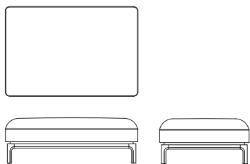
ワイド 2P ベンチ X02640S 【 W1245 D845 H425 】
