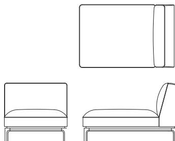
肘無シェーズロング L09130N 【W820 D1235 H765 SH425】
