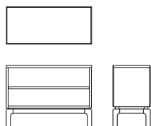
シェルフ B09170Z 【 W800 D350 H590 】
