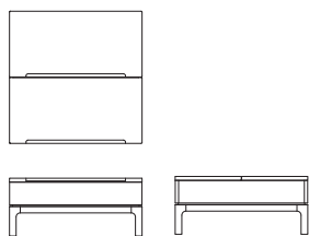
リビングテーブル T04780Y 【W800 D800 H350】
