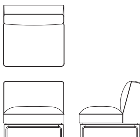
肘無 1P ソファ L09110N 【W820 D835 H765 SH425】
