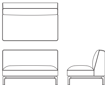
肘無ワイド 2P ソファ L09110F 【W1220 D835 H765 SH425】
