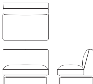
肘無 2P ソファ L09110D 【W1020 D835 H765 SH425】
