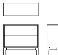
シェルフ B09161Z 【 W800 D290 H720 】
