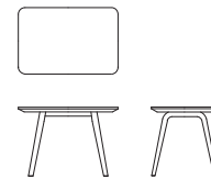
1P スツール X02610Z 【W600 D400 H415】
