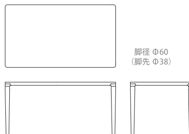
ダイニングテーブル R03970C 【 W1500(1380) D850(730) H720 】
