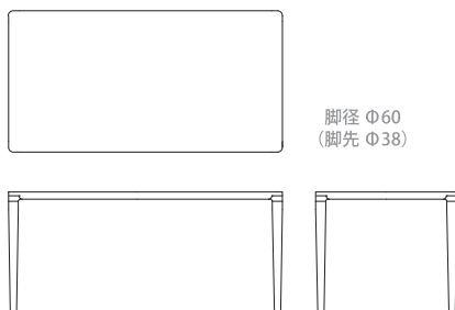
ダイニングテーブル R03970X 【 W1650(1530) D850(730) H720 】
