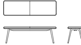
ワイド2Pベンチ X02611F WN [W/1400 D/400 H/445]
