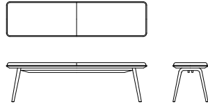
3Pベンチ X02611S WN [W/1600 D/400 H/445]
