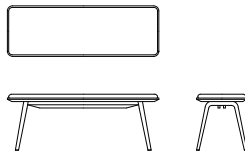
2Pベンチ X02611D WN [W/1200 D/400 H/445]
