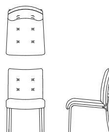
アームレスチェア D04210N [W/520 D/635 H/860 SH/450]
