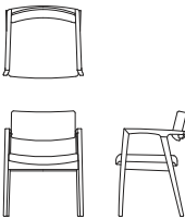
ワイドアームチェア D03780B OIL WN [W/580 D/525 H/765 SH/435 AH/640]
